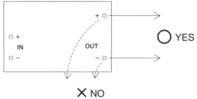
Fig.5.1 Pattern wiring
